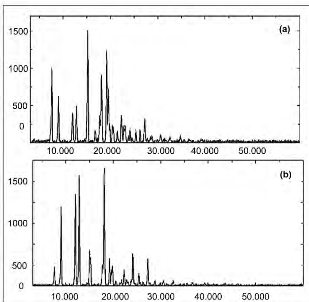
Figura 27. Espectros obtidos em análises por difração de Raios X das amostras Y1 (a) e Y2 (b).
