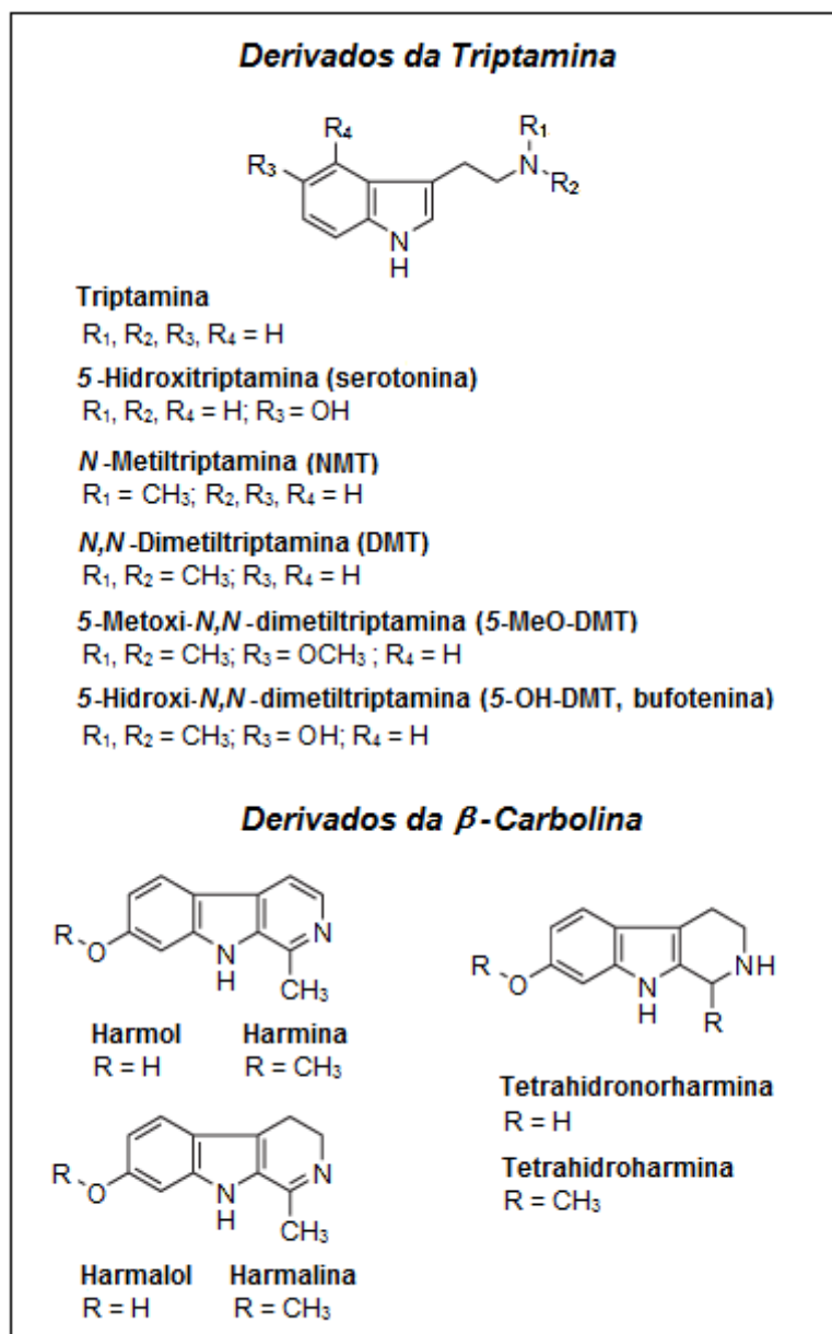
Figura 3. Estruturas gerais para os derivados da triptamina e da \beta -carbolina.
