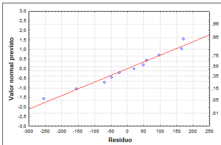
Figura 37. Gráfico de probabilidade normal para o modelo quadrático.
