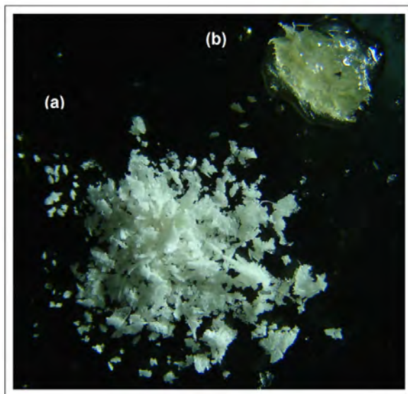
Figura 11. Fotografia das frações branca e amarela de N,N -dimetiltryptamina, isolado das cascas de M. tenuiflora . (a) Fração branca e (b) fração amarela. Foto: Alain Gaujac
